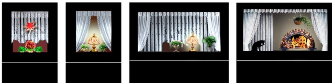
LD041/nw LD042/ww LD043/ww LD044/ww Abmessung: Träger BxH 16x18 / 29x18 mm / Fenster BxH 10x12 / 24x12 mm / Leuchtfläche: bis Fensterfläche LED normalweiß / warmweiß / 5,6k - 1,5 mA
